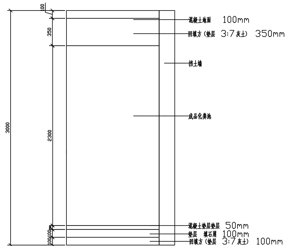
化粪池剖面图
